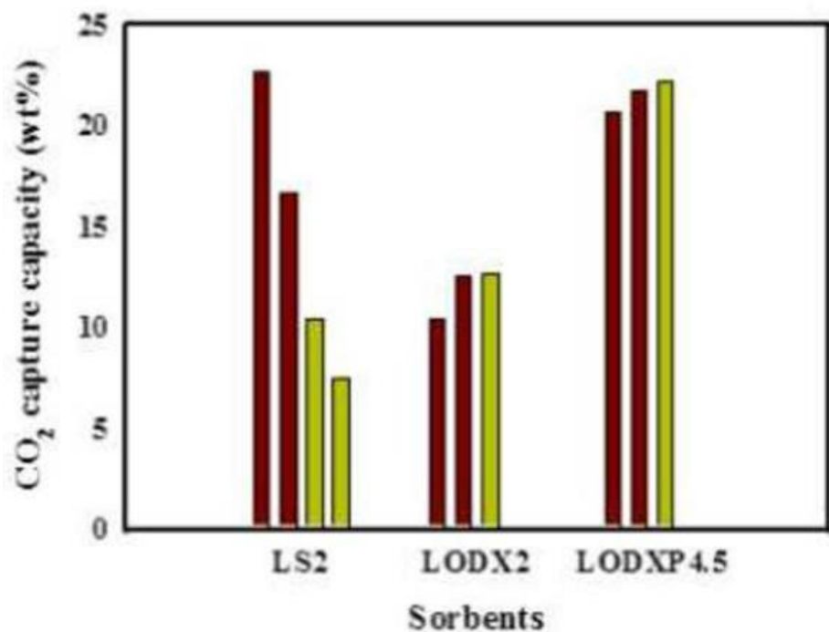
<이산화탄소 흡수능 측정결과>
