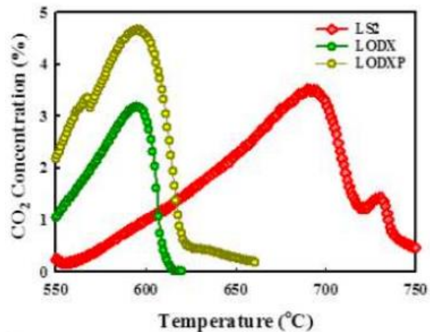
<흡수체의 TPD 분석결과>
